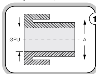
disegno dimensionale / reference details
