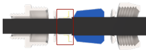
Esplora vista pressacavo EMC non armato Explore view EMC non-armoured cable gland
